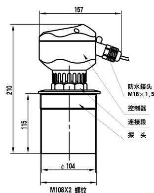
M108×2 螺纹传感器
