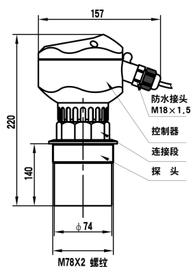
M78×2 螺纹传感器
