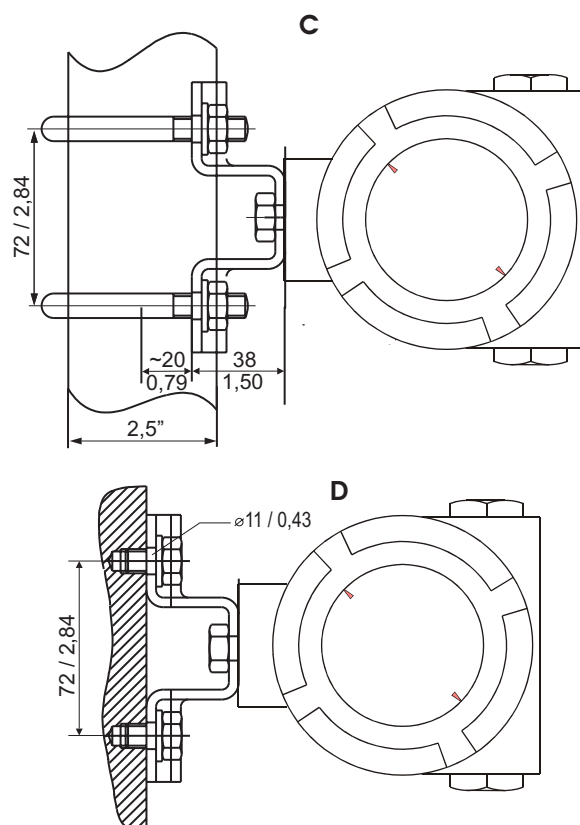
C 管道安装 D 墙壁安装
